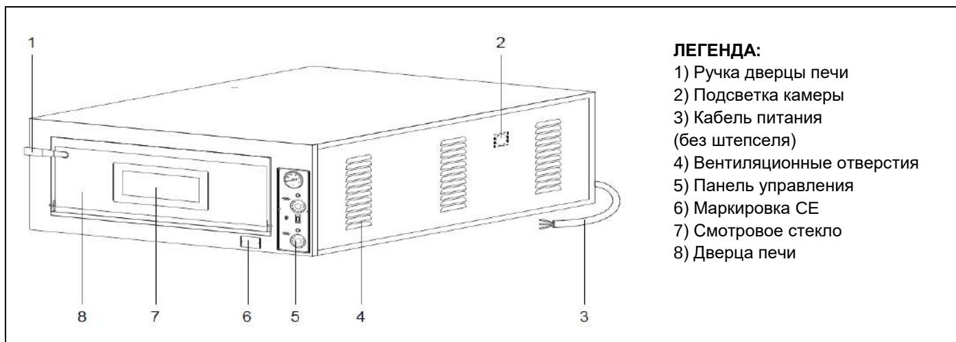
РИС.2 (Наименование составных частей)
