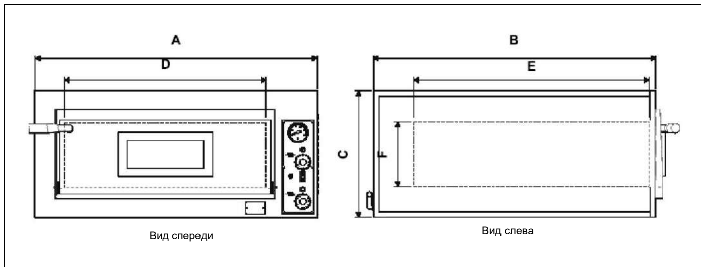
РИС.3 (Размеры печи и выпечной камеры)
