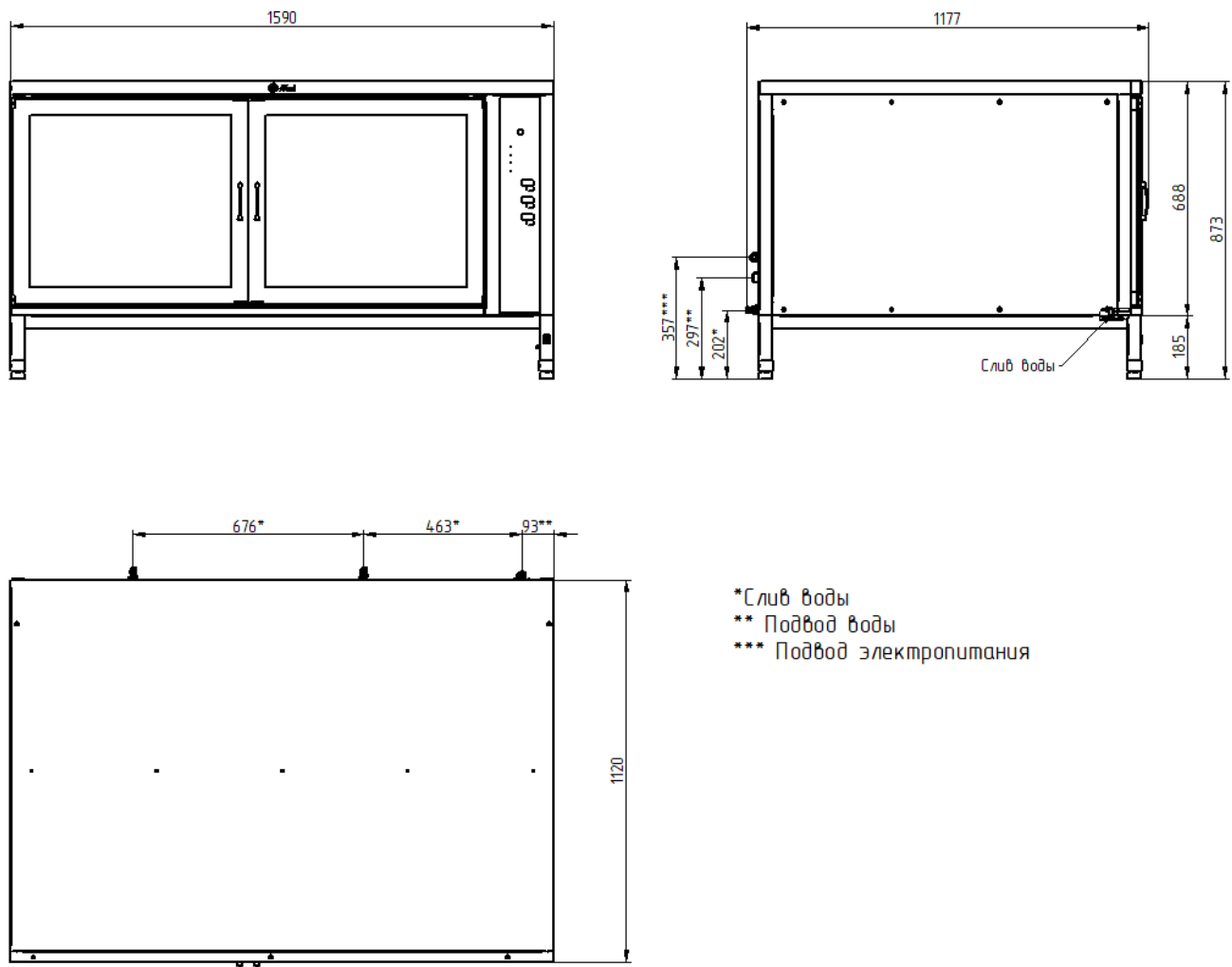
Рис.1 Шкаф расстоечный тепловой ШРТ-6-ЭШП-4EN-Super.
