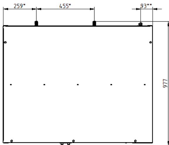
Рис.1 Шкаф расстоечный тепловой ШРТ-6-ЭШП-2EN-Super.
