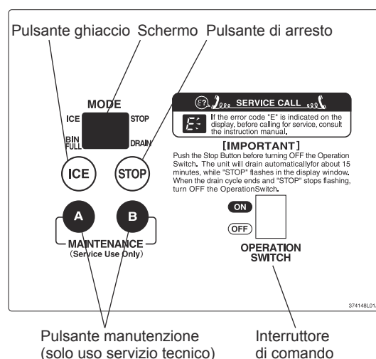
Pannello di comando
